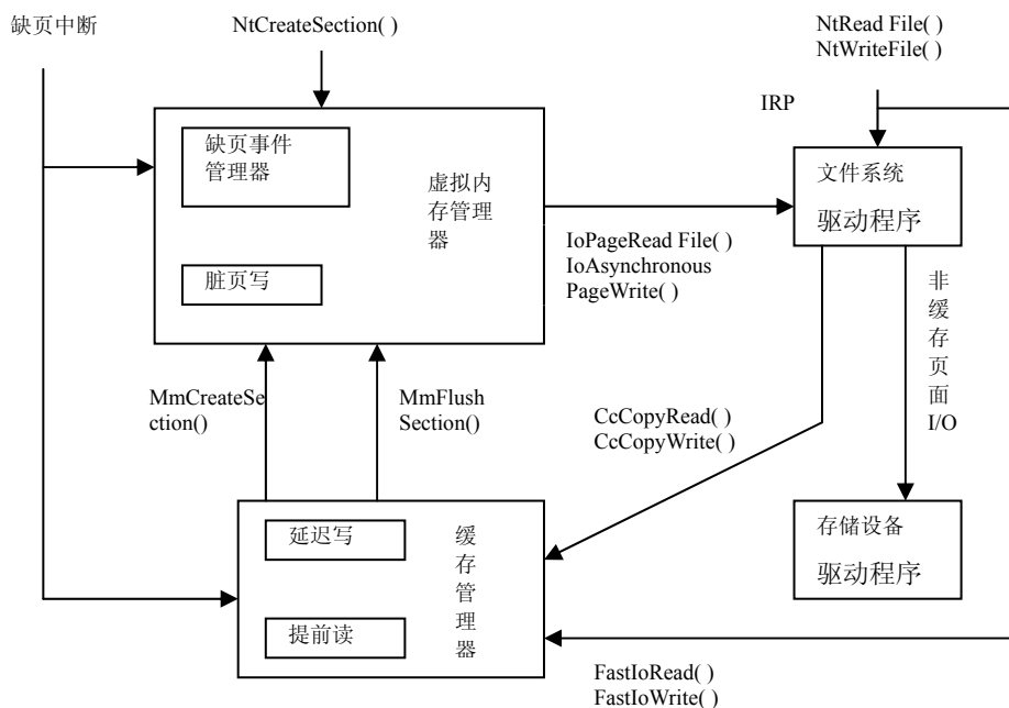
图 6-27 FSD 的作用
