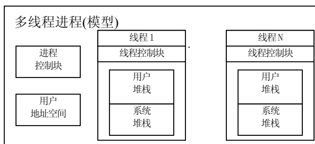
图 2-27 多线程进程
