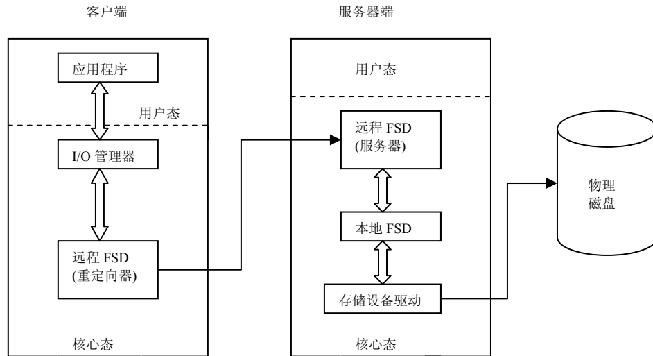
图 6-26 远程 FSD
