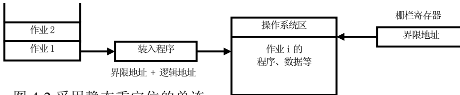
图 4-2 采用静态重定位的单连
