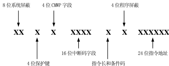
图 2-1 IBM 370 系统程序状态字的基本控制格式
