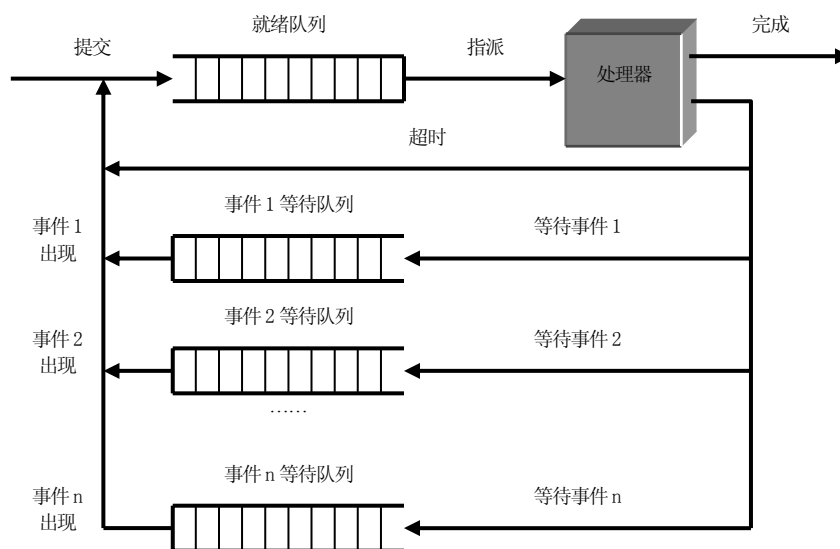
图 2-20 操作系统的队列管理和状
