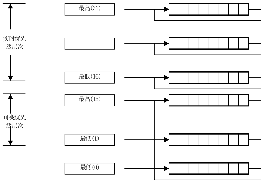
图 2-43 Windows 2000/XP 线程优先级
