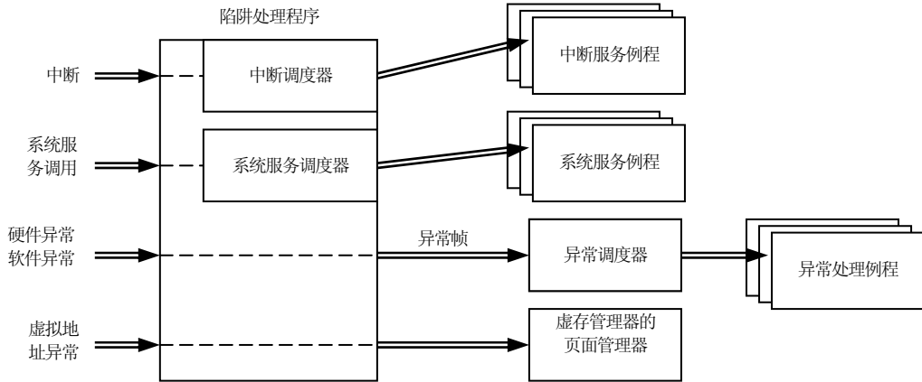
图 2-7 Windows2000/XP
