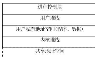
图 1-13 OS 的所有功能（函数）在用户进程内执行模型的进程映像
