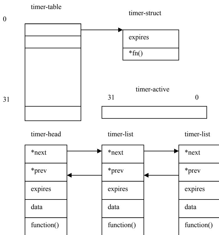
图 2-6 系统计时器
