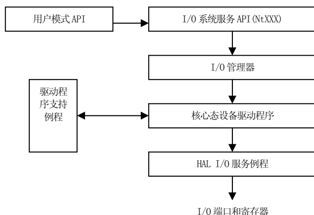
图 5-13 一个典型的 I/O 请求流程
