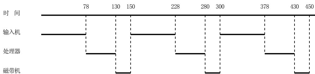
图 1-3 单道算题运行时处理器的使用效率
