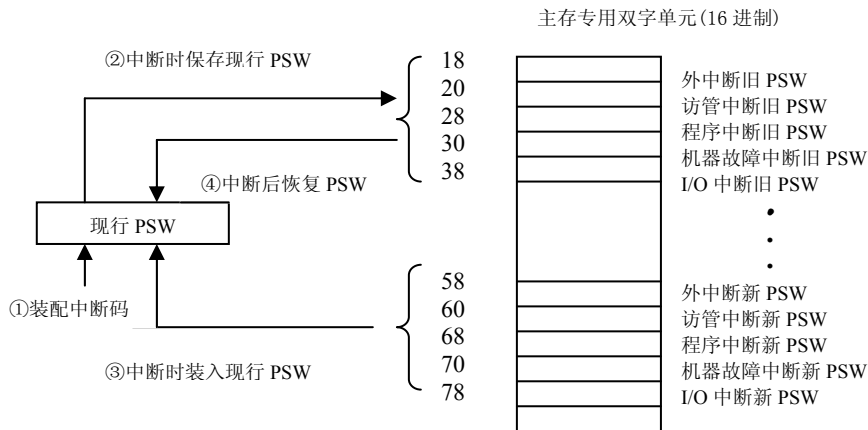
图 2-3 IBM 中大型机中断响应过程
