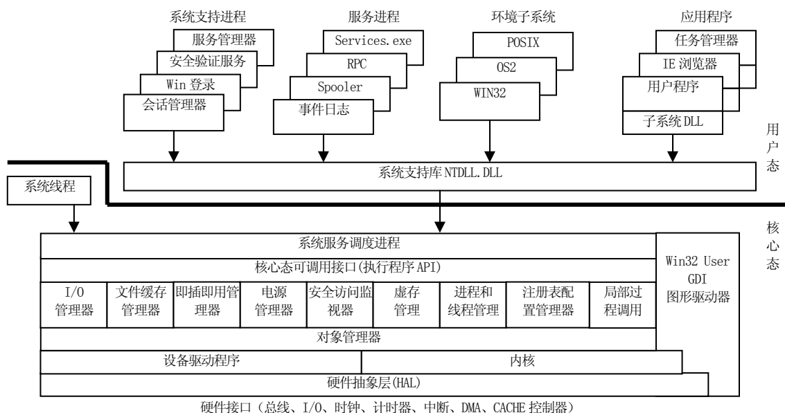
图 1-15 Windows 2000/XP
