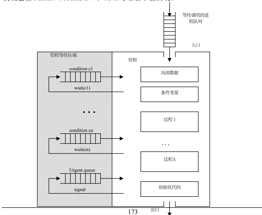
图 3-5 管程的结构示意图
