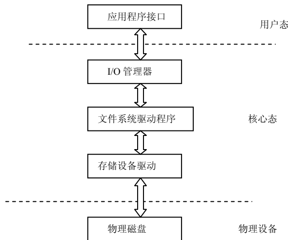
图 6-25 本地 FSD
