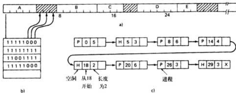
图 4-14 内存分配的位示图和链表方法
